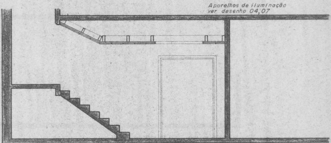
SEÇÃO C-D
