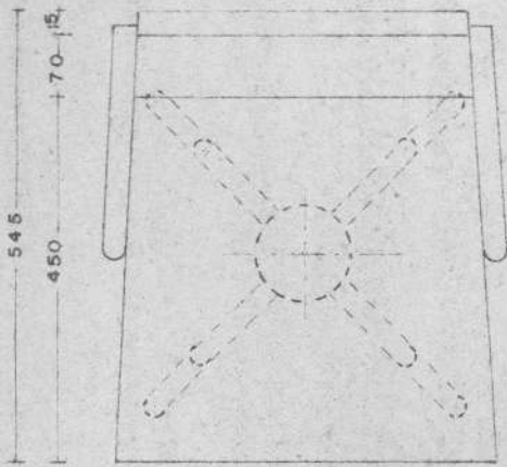
PLANTA SEM ESTOFO
