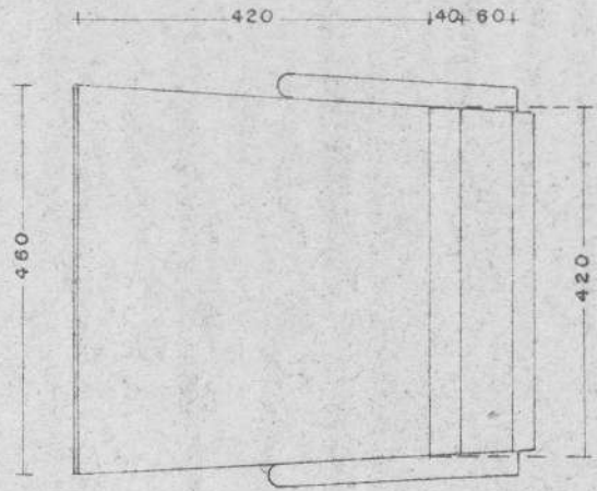
PLANTA COM ESTOFO
