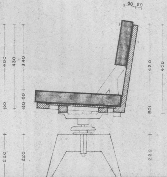
CORTE
