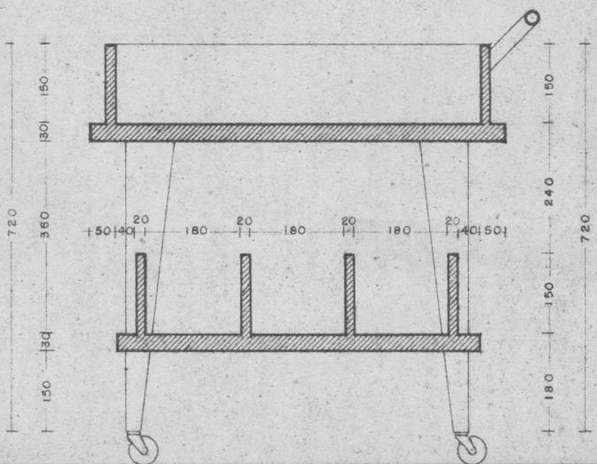
CORTE
