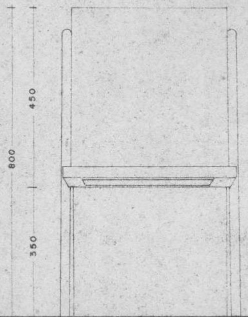
VISTA DE FRENTE SEM ESTOFO
