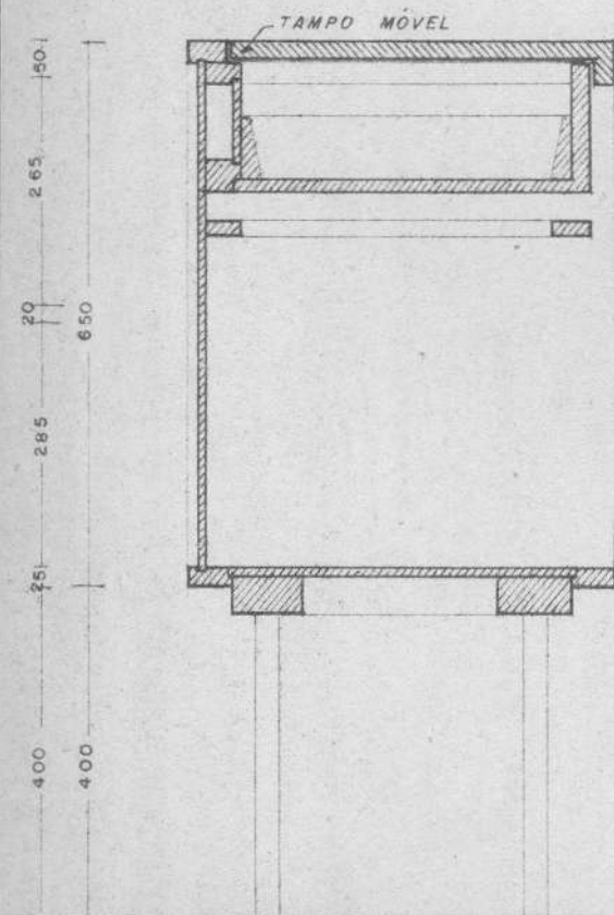
SEÇÃO B B
