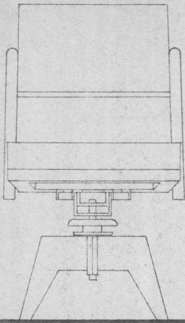
VISTA DE FRENTE
